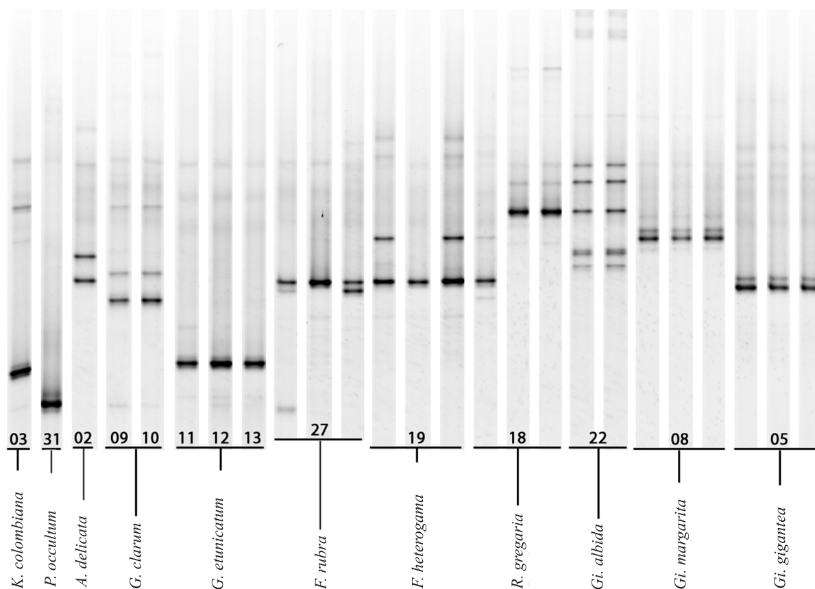
Figura 2. Perfis de DGGE da região V9 da subunidade menor do gene ribossômico (18S rRNA), dos 14 isolados da coleção de FMA utilizada.
