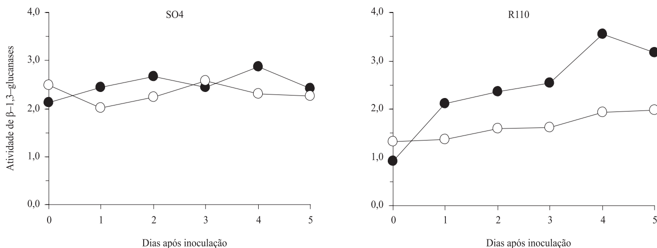
Figura 2. Atividade de \beta -1,3-glucanases (unidades de absorbância a UA 600 nm por miligrama de proteína por hora), em amostras radiculares de porta-enxertos de videira – suscetível (SO4) e resistente (R110) a Fusarium oxysporum f. sp. herbemontis coletadas entre um e cinco dias após a inoculação do patógeno (—●—) ou a imersão de raízes em água estéril (—○—).
