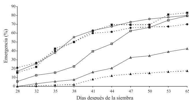
Figura 2. Emergencia de plántulas de Mandarino 'Cleopatra' en Cazonos, Veracruz, a partir de semillas almacenadas durante seis meses, con 26,8% (■ y □), 14,7% (▲ y △) y 5% (● y ○) de humedad, sin 8-hidroxiqinoleina (---) y con 8-hidroxiqinoleina (—).
