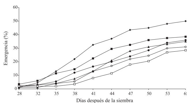
Figura 1. Emergencia de plántulas de Mandarina 'Cleopatra' en Cazonos, Veracruz, a partir de semillas almacenadas durante seis meses, tratadas con 8-hidroxiquinoleina (◆), Rodamina (■), Tecto 60 (▲), Captan (●), Interguzan (○) y Testigo (□).
