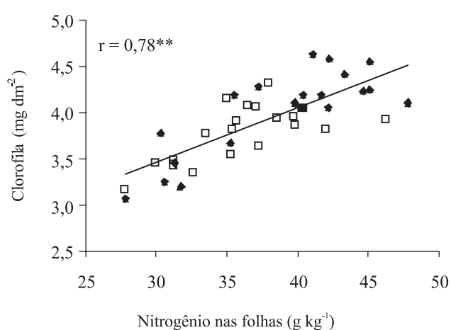
Figura 2. Correlação entre teor de clorofila e de nitrogênio nas folhas do feijoeiro, em sistema de plantio direto ( \square ) e preparo convencional do solo ( \blacklozenge ). **Significativo a 1% de probabilidade pelo teste t.
