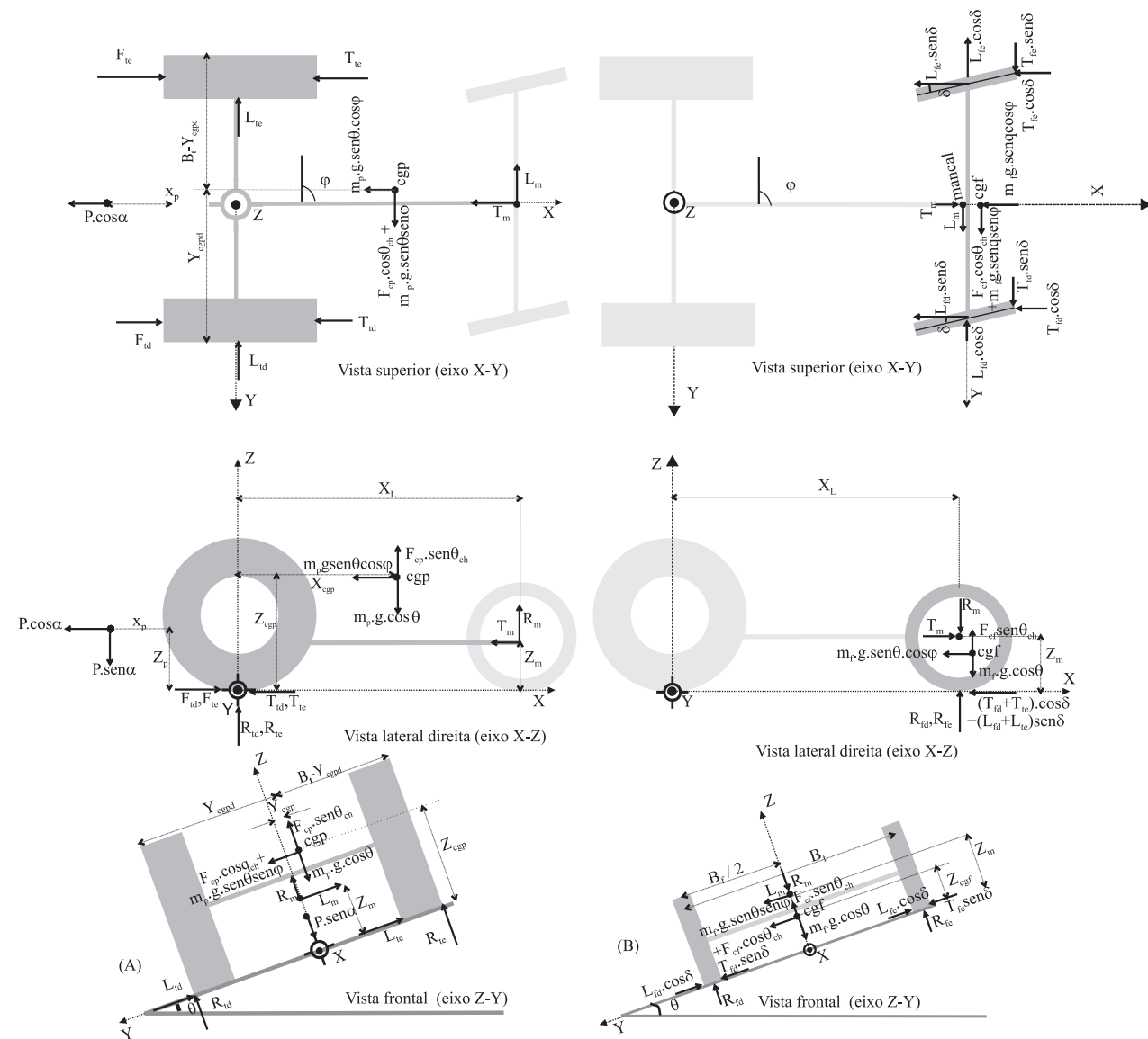
Figura 3. Diagrama de corpo livre da massa parcial (A) e eixo frontal (B) do trator, com vistas superior, lateral direita e frontal.
