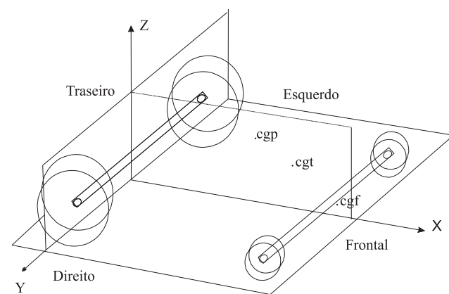
Figura 1. Sistema de coordenadas para localização dos centros de gravidade parcial (cgp), total (cgt) e frontal (cgf).
