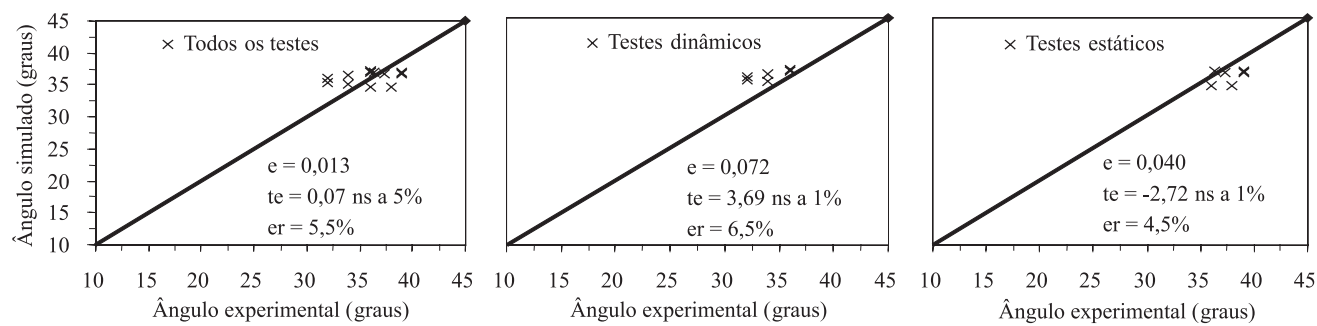
Figura 4. Gráfico de correspondência de inclinação de tombamento entre os valores experimentais e simulados, mostrando o erro relativo médio (e) e o erro relativo absoluto médio (er) entre o valor simulado e o experimental e o teste estatístico t do erro e (te).
