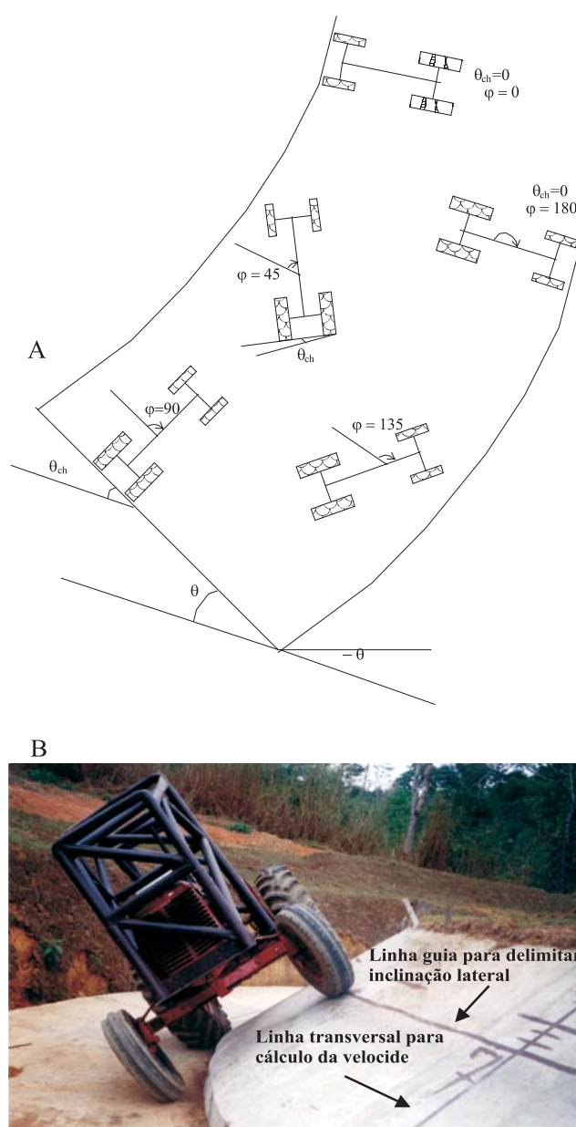
Figura 2. A: esquema de algumas orientações do trator operando em uma pista inclinada; B: vista frontal do trator, fazendo curva em pista inclinada, em curva de nível, a uma velocidade constante e ângulo \varphi = 90^\circ (B) (Khoury Junior et al., 2001).
