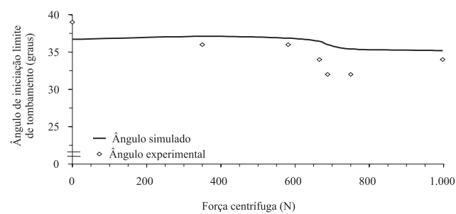
Figura 5. Ângulo de inclinação do limite de tombamento em função da força centrífuga calculada.
