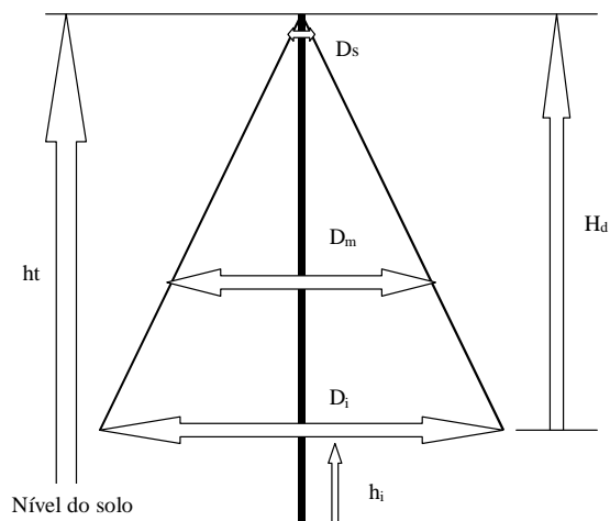
Figura 1. Variáveis de arquitetura de parte aérea da planta de café: ht: altura (m) da planta, Hd: altura (m) do dossel, hi: altura (m) de inserção do primeiro par de ramos plagiométricos, Di: diâmetro (m) da seção inferior do dossel, Dm: diâmetro (m) da seção média do dossel, e Ds: diâmetro (m) da seção superior do dossel.
