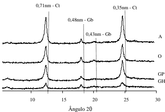
Figura 1. Difratogramas de raios X da fração argila desferificada, saturada com sódio, à temperatura ambiente e lâminas orientadas, no horizonte A dos solos de várzea. Caulinita (Ct), gibbsita (Gb), Aluvial (A), Glei Pouco Húmico (GP), Glei Húmico (GH) e Orgânico (O).
