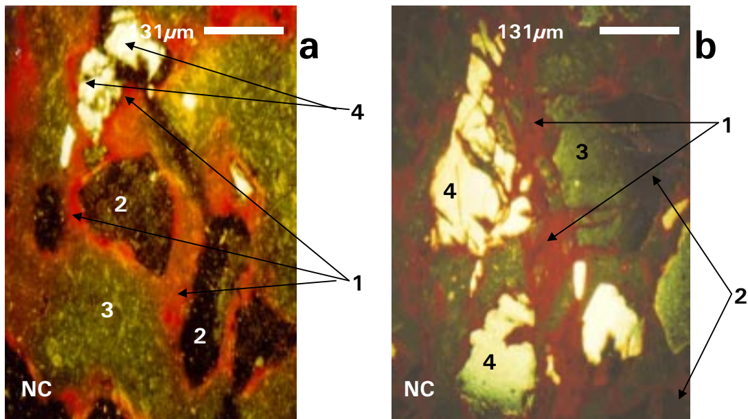
FIG. 5. Micrografias de áreas de mosqueado do Plintossolo (P26) a duas profundidades: a) 150 cm de profundidade, presença de ferrões com camada difusa; b) 300 cm de profundidade, ferrões sem camada difusa: 1 - ferrões; 2 - poros; 3 - matriz caulínica; 4 - grãos de quartzo. NC: nicóis cruzados.
