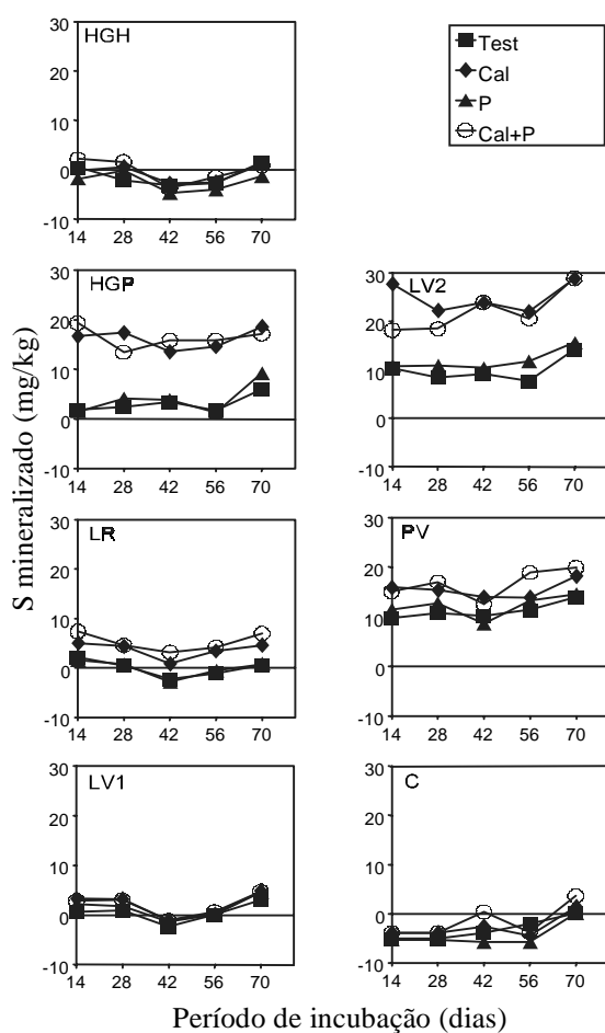
FIG. 3. Mineralização líquida de enxofre, ao término dos cinco períodos de incubação, sob influência da calagem e da adição de fósforo. HGH: Gleí Húmico; HGP: Gleí Pouco Húmico; LR: Latossolo Roxo; LV1: Latossolo Vermelho-Amarelo (Itumirim); LV2: Latossolo Vermelho-Amarelo (Rio de Janeiro); PV: Podzólico Vermelho-Amarelo; C: Cambissolo.
