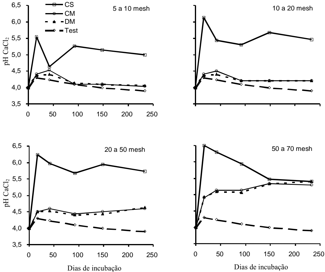
FIG. 2. Efeito da aplicação de calcários calcítico sedimentar (CS), calcítico metamórfico (CM) e dolomítico metamórfico (DM) em diferentes granulometrias (peneiras de 5 a 10, 10 a 20, 20 a 50 e 50 a 70 mesh), sobre o pH de um Latossolo Roxo (LRd) após incubação ao longo de 233 dias (testemunha sem calcário = Test).
