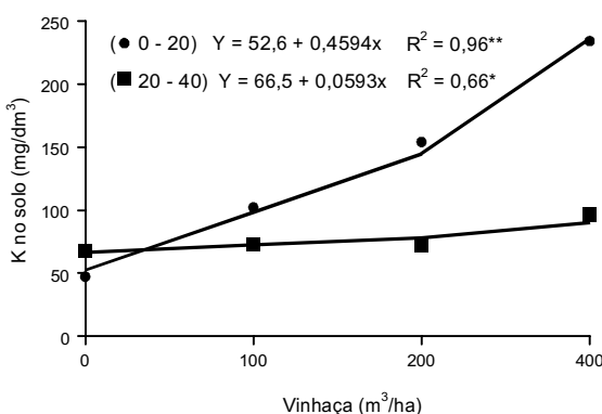
FIG. 5. Efeito das doses de vinhaça sobre os teores de K no solo à profundidade de 0-20 e 20-40 cm.
