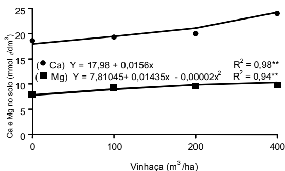
FIG. 6. Efeito das doses de vinhaça sobre os teores de Ca e Mg no solo, à profundidade de 0-20 cm.
