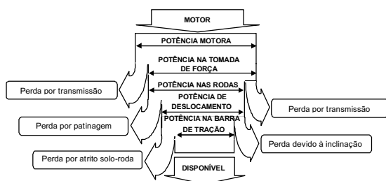
FIG. 3. Esquema da distribuição de uso de potência do trator e suas perdas. Fonte: Piroi & Vaitilangom (1987).
