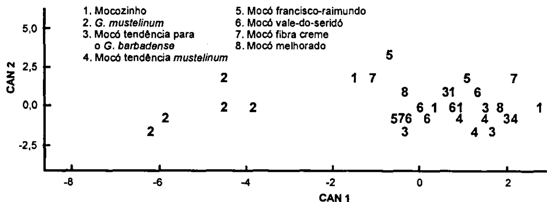
FIG. 3. Distribuição dos pontos correspondentes aos algodoeiros nos primeiro e segundo eixos canônicos.
