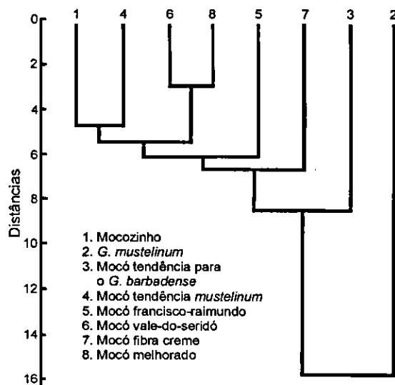
FIG. 1. Dendrograma resultante da classificação dos algodoeiros pela análise de conglomerados.
