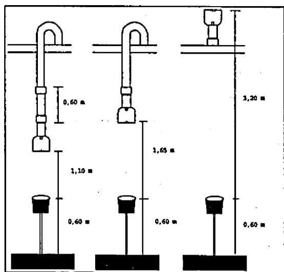
FIG. 2. Ilustração da posição dos emissores.
