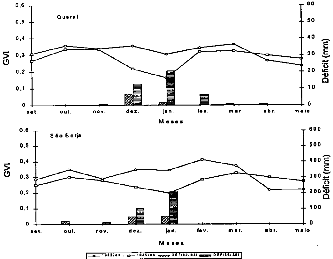
FIG. 4. Índice de vegetação global (GVI) e déficit hídrico em Quarai e São Borja, período 1982/86.
