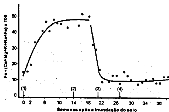
FIG. 1. Relação Fe \div (Ca + Mg + K + Na + Fe) \times 100 em solo Gley Pouco Húmico durante a inundação e após a drenagem: (1) início da inundação; (2) início da drenagem; (3) fim da drenagem; (4) plantio do feijão (Moraes & Dynia, 1992).
