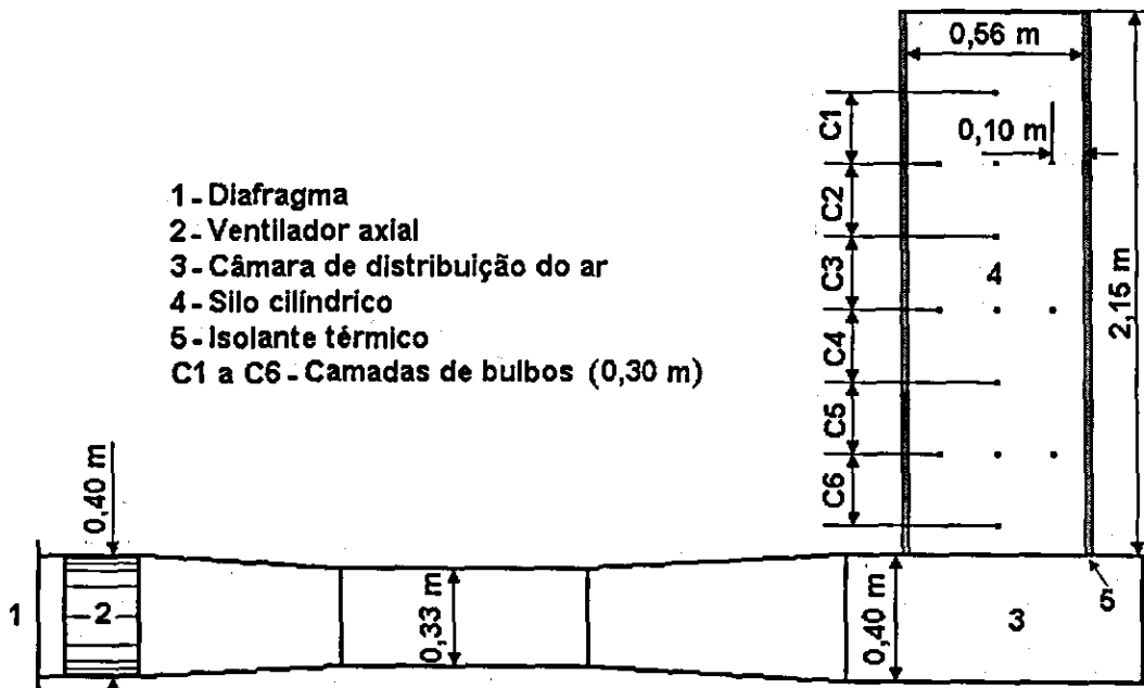
FIG. 1. Vista lateral do silo de aeração.
