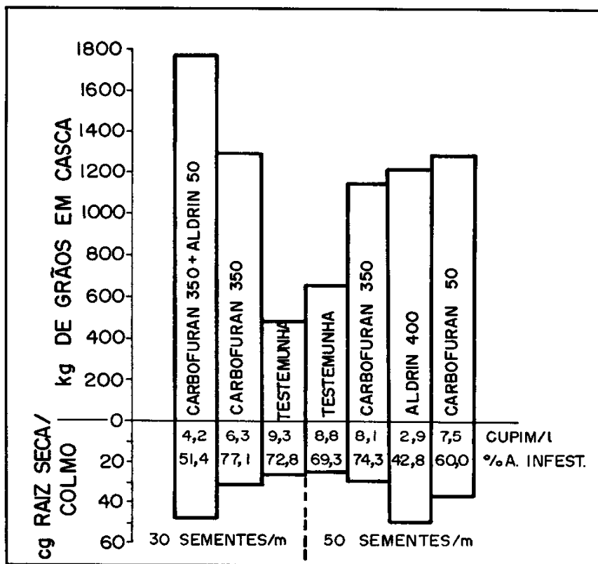
FIG. 1. Influência da densidade de semeadura e tratamentos sobre cupim, peso seco das raízes e rendimento de grãos. Santo Antônio de Goiás, GO, 1983/84.
