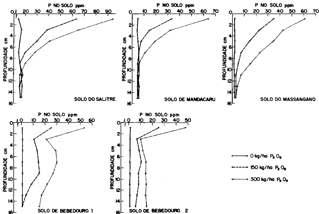
FIG. 1 - Movimento do fósforo aplicado na superfície (0-2 cm) de cinco solos acondicionados em colunas lixivia-doras.
