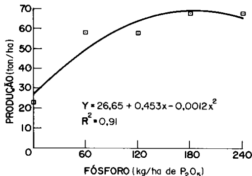
FIG. 2 - Resposta do tomateiro à adubação fosfatada.
