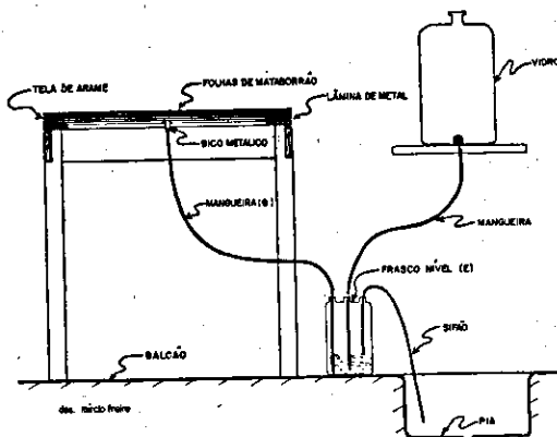
FIG. 1. Desenho em corte do aparelho "mesa de tensão" (segundo Leamer & Shaw 1941).
