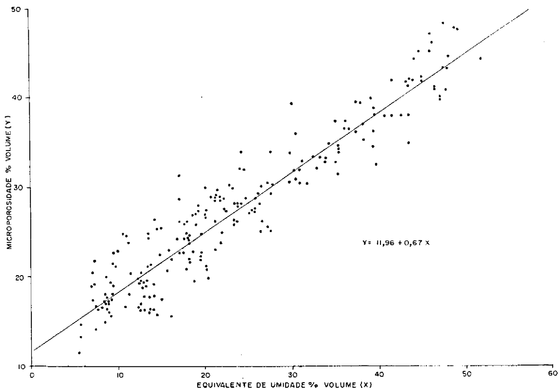
FIG. 1. Retã e equaão de regressão do estudo de correlaão entre o equivalente de umidade e a microporosidade em solos podzolizados no Nordeste do Brasil.
