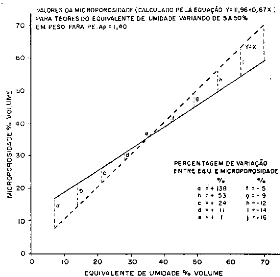
FIG. 2. Diferenas e percentagens de variaão entre os valores do equivalente de umidade ( Y = X ) e da microporosidade calculada ( Y = 11,96 + 0,67 X ) numa faixa de valores entre 5 e 50% para Eq.U, expressos em % peso.
