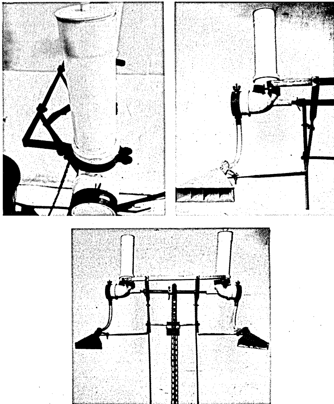
FIG. 7. Ilustrações dos detalhes de acoplamento das peças que compõem o sistema de suporte, distribuição e transmissão da rotação do implemento para a aplicação do inseticida.
