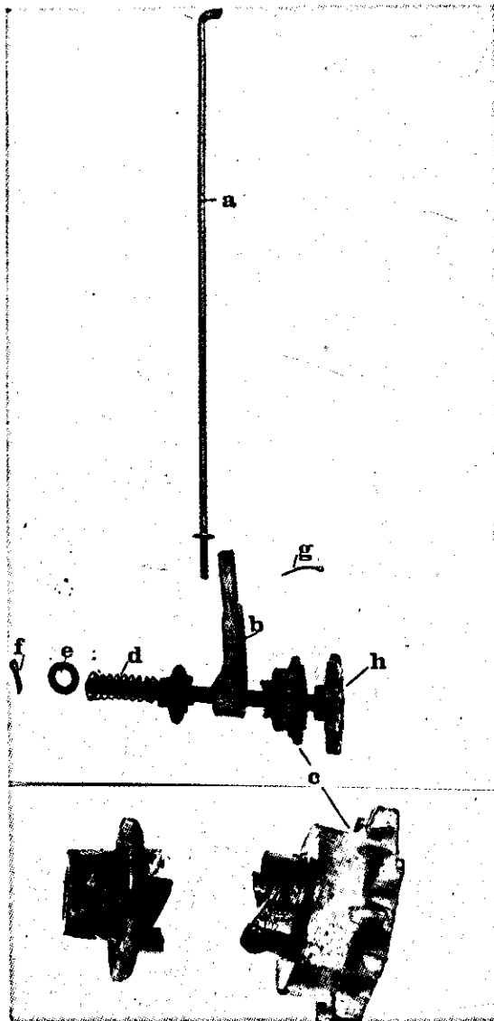
FIG. 2. Sistema de engate para acionar ou desligar a saída do inseticida montado sobre o eixo inferior do implemento. (a) cabo; (b) separador; (c) catracas; (d) mola; (e) arruela; (f) contrapino da mola; (g) contrapino do cabo; (h) engrenagem do eixo.
