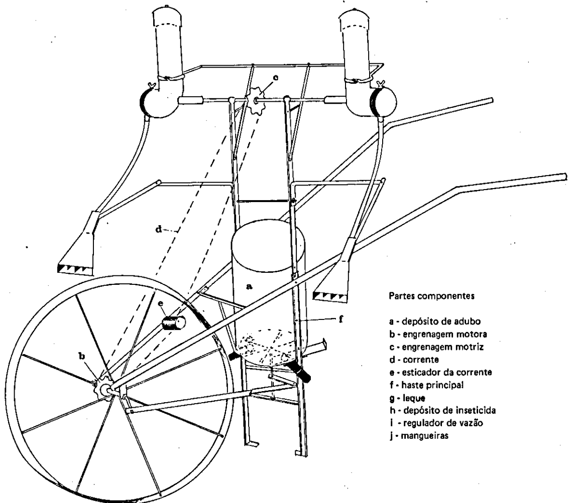
FIG. 8. Desenho esquemático do implemento para aplicação de inseticida granulado diretamente no cartucho das plantas de milho ou de sorgo, adaptado a adubadeira manual.
