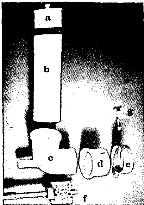
FIG. 5. Detalhe da montagem do implemento para aplicação do inseticida granulado. (a) tampão; (b) depósito do inseticida; (c) curva (joelho); (d) tubo; (e) anel de metal; (f) escova e (g) parafuso, arruela e "borboleta".
