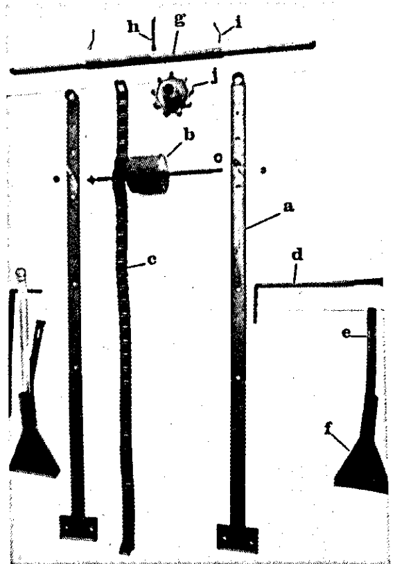
FIG. 3. Adaptações necessárias ao funcionamento do implemento para aplicação de inseticidas granulados. (a) suporte vertical do mecanismo de distribuição do inseticida; (b) esticador de corrente; (c) corrente; (d) braços laterais; (e) suporte do leque de distribuição do inseticida; (f) leque de distribuição do inseticida; (g) eixo superior; (h) contra-pino da catraca; (i) contra-pino do eixo e (j) catraca.
