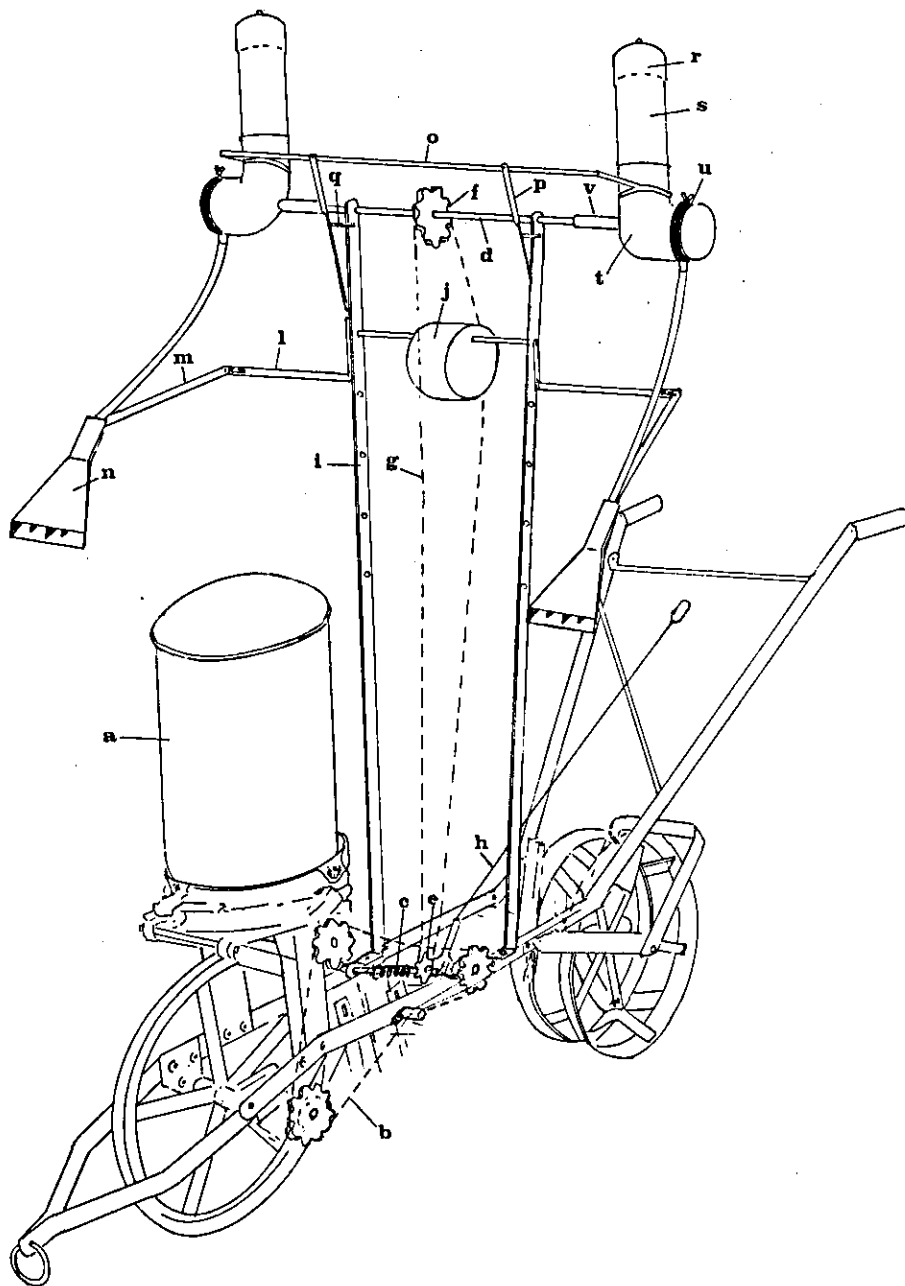
FIG. 1. Desenho esquemático do implemento para aplicação de inseticida granulado diretamente no cartucho das plantas de milho ou de sorgo, adaptado à plantadeira de tração animal. (a) - Depósito de adubo; (b-g) - corrente; (c-d) - eixo; (e-f) - engrenagem; (h) - alavanca para acionar o sistema; (i-m-l-o-p) - hastes; (j) esticador; (n) - leque; (q) suporte de haste; (r) - tampa do depósito de inseticida; (s-t) - depósito de inseticida; (u) - regulador de vazão.
