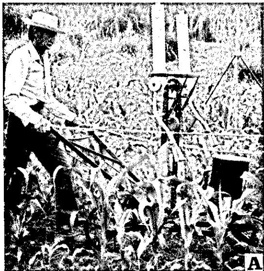
FIG. 9. Implemento para aplicação de inseticida granulado diretamente no cartucho de plantas de milho e sorgo e para aplicação de adubo nitrogenado em cobertura. (a) tração animal; (b) manual.
