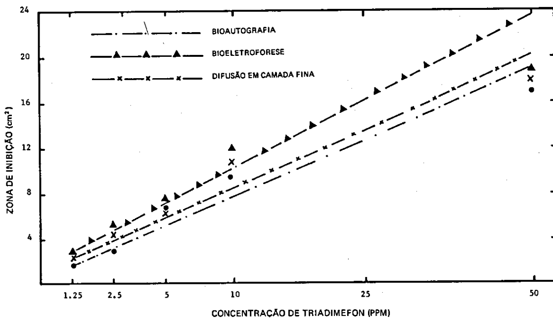
FIG. 5. Relação semilogarítmica entre a área da zona de inibição do crescimento de Thielaviopsis paradoxa e a concentração de triadimefon aplicada.
