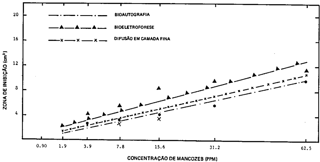
FIG. 7. Relação semilogarítmica entre a área da zona de inibição do crescimento de Thialaviopsis paradoxa e a concentração da mancozeb aplicada.
