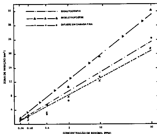
FIG. 4. Relação semilogarítmica entre a área da zona de inibição do crescimento de Thielaviopsis paradoxa e a concentração de benomil aplicada.
