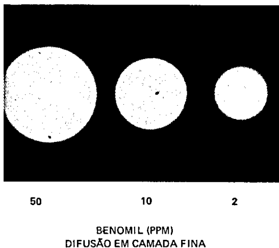
FIG. 1. Difusão em camada fina de concentrações crescentes de benomil com Thielaviopsis paradoxa como organismo-teste.
