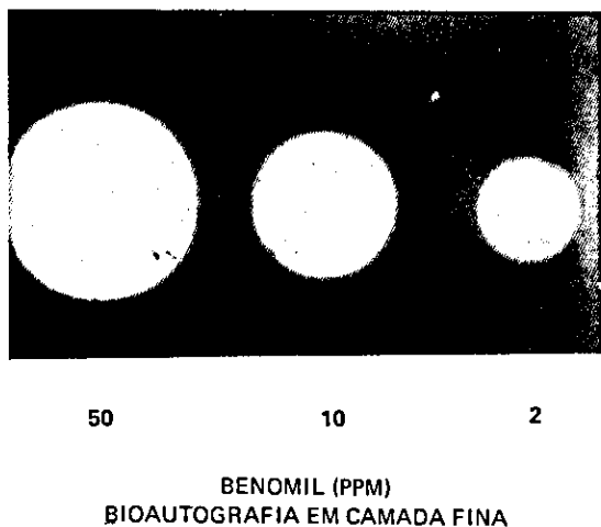
FIG. 2. Bioautografia em camada fina de concentrações crescentes de benomil com Thielaviopsis paradoxa como organismo-teste.
