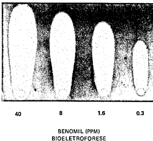
FIG. 3. Bioeletroforese de concentrações crescentes de benomil com Thielaviopsis paradoxa como organismo-teste.
