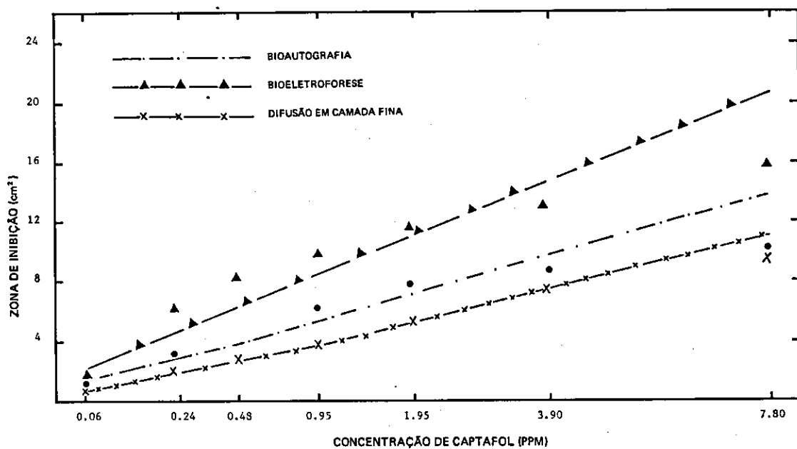
FIG. 6. Relação semilogarítmica entre a área da zona de inibição do crescimento de Thielaviopsis paradoxa e a concentração de captafol aplicada.
