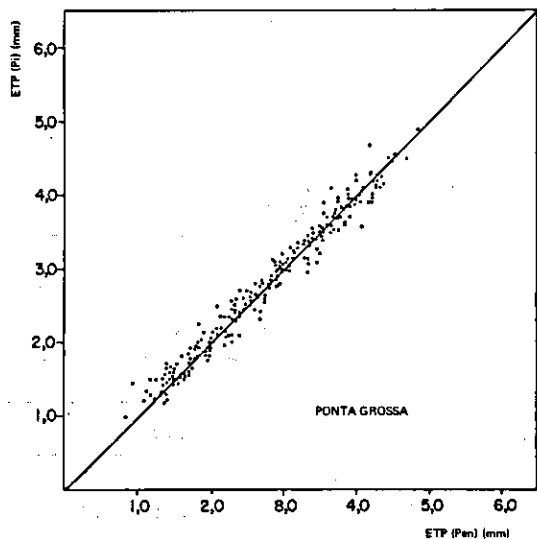
FIG. 2. Relação entre os valores de evapotranspiração calculados pelo método original de Penman (ET o Pen) e o método simplificado (ET o Pi), para Ponta Grossa, PR.
