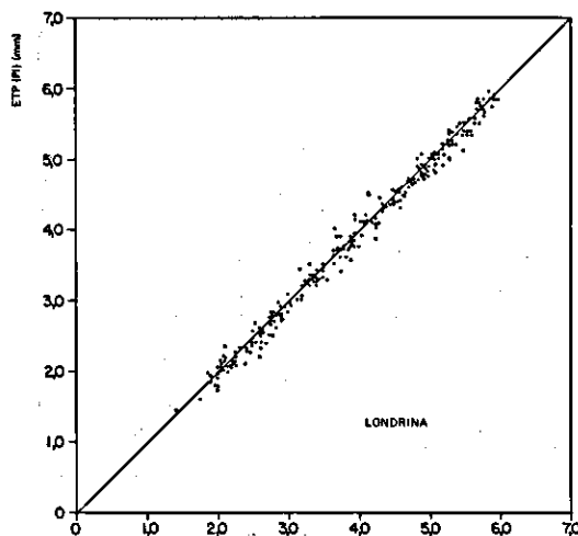
FIG. 1. Relação entre os valores de evapotranspiração calculados pelo método original de Penman (ET o Pen) e o método simplificado (ET o Pi), para Londrina, PR.
