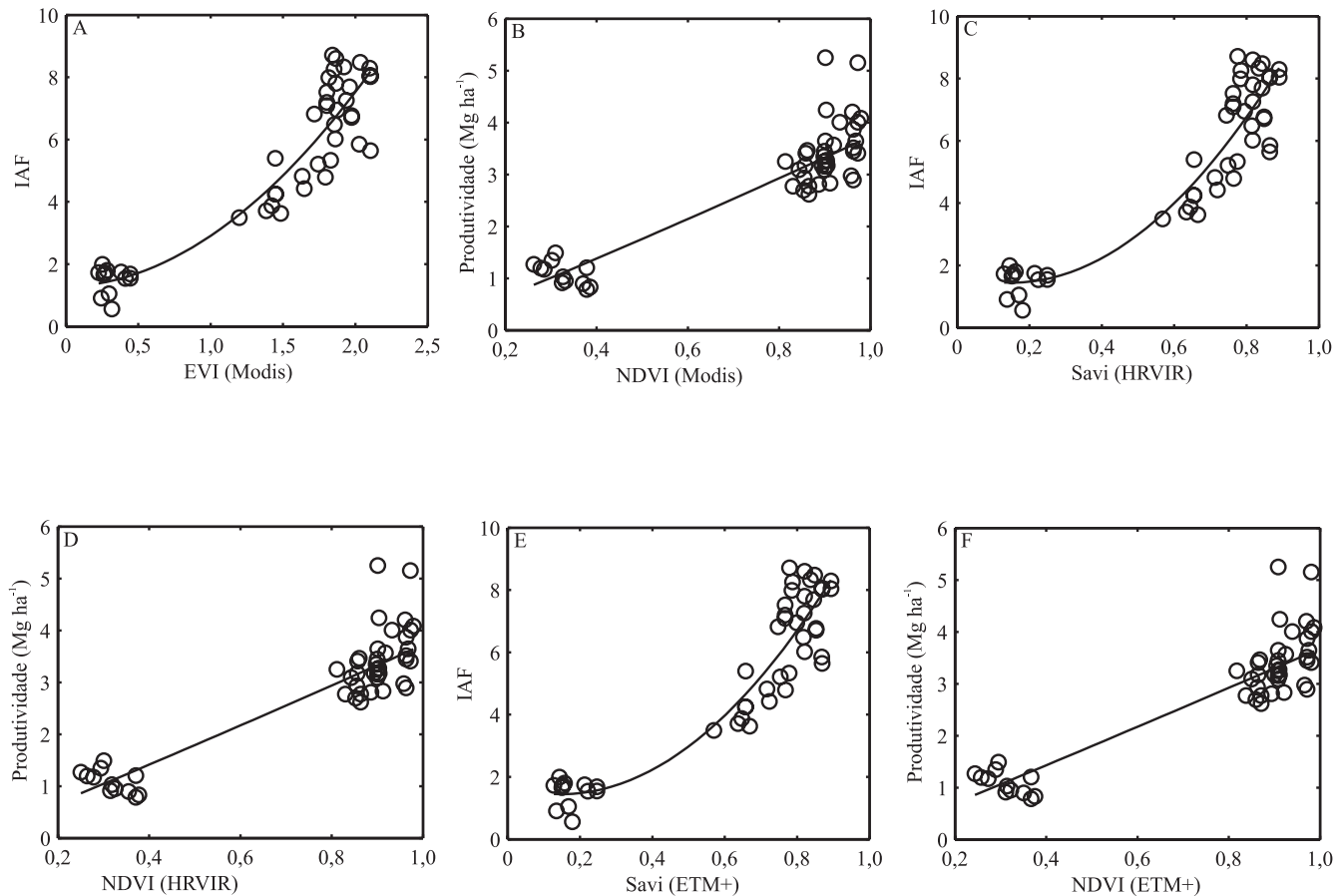
Figura 2. Diagramas de dispersão entre as variáveis biofísicas e os índices de vegetação mais bem ajustados dos sensores analisados no estádio R6 da cultura do feijoeiro. A, índice de área foliar (IAF) e EVI (Modis); B, produtividade e NDVI (Modis); C, IAF e Savi (HRVIR); D, produtividade e NDVI (HRVIR); E, IAF e Savi (ETM+); e F, produtividade e NDVI (ETM+).
