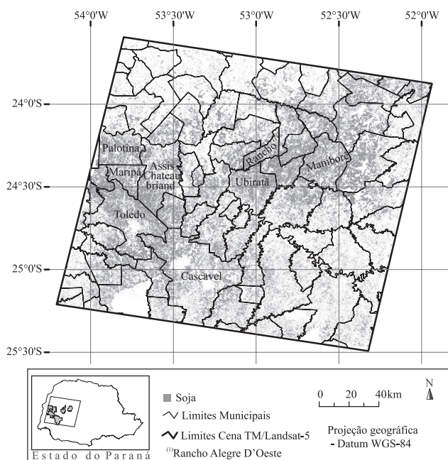
Figura 1. Máscara de soja gerada a partir da classificação de imagens TM/Landsat-5, para oito municípios do Estado do Paraná, com dados referentes à safra de 2003/2004.
