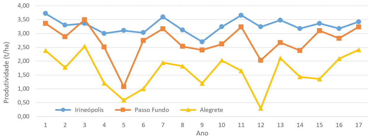
Figura 2. Produtividades municipais de soja entre 2001 e 2017, com tendência removida, nos municípios de Irineópolis em Santa Catarina, Passo Fundo e Alegrete no Rio Grande do Sul.
