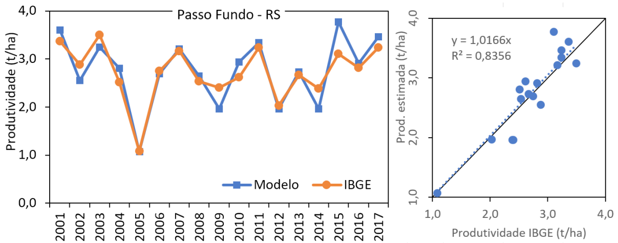
Figura 3. Séries de produtividade de soja entre 2001 e 2017 levantadas pelo IBGE, com tendência removida, e séries de produtividade estimadas pelo modelo de produtividade baseado em disponibilidade hídrica.
