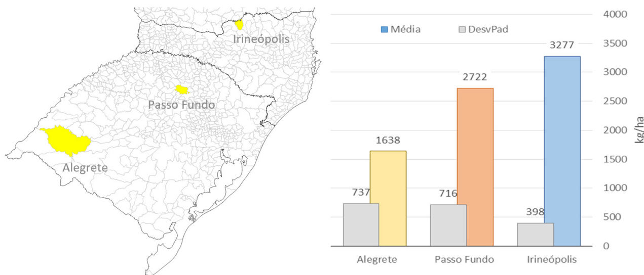
Figura 1. Localização e produtividades médias de soja e desvio padrão entre 2001 e 2017 dos municípios de Irineópolis em Santa Catarina, Passo Fundo e Alegrete no Rio Grande do Sul.
