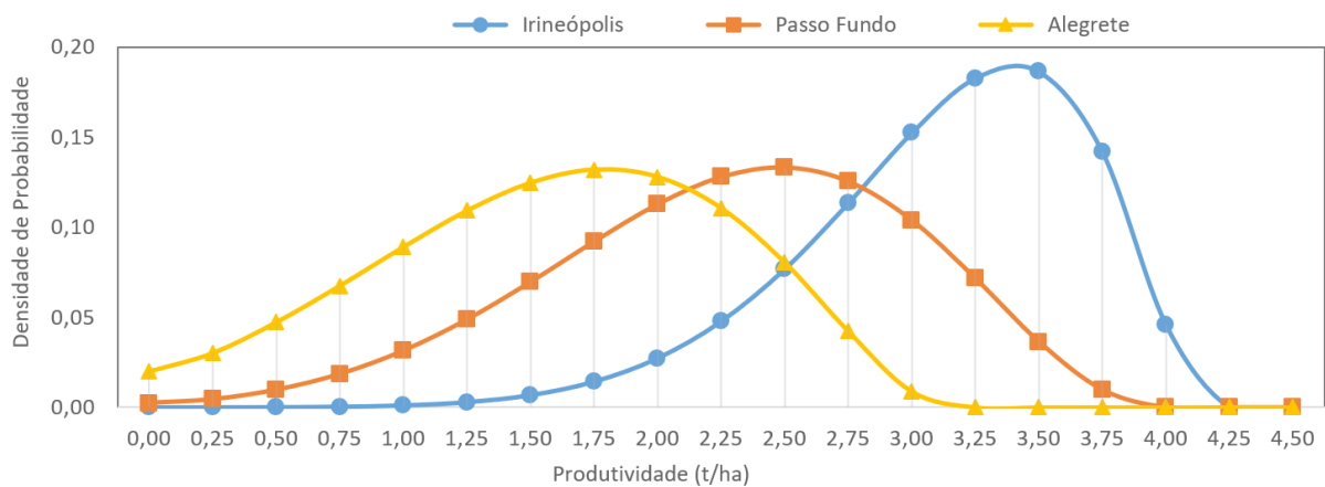
Figura 4. Distribuição Beta de frequência ajustada das séries de produtividade de soja entre 2001 e 2017, nos municípios de Irineópolis em Santa Catarina, Passo Fundo e Alegrete no Rio Grande do Sul.
