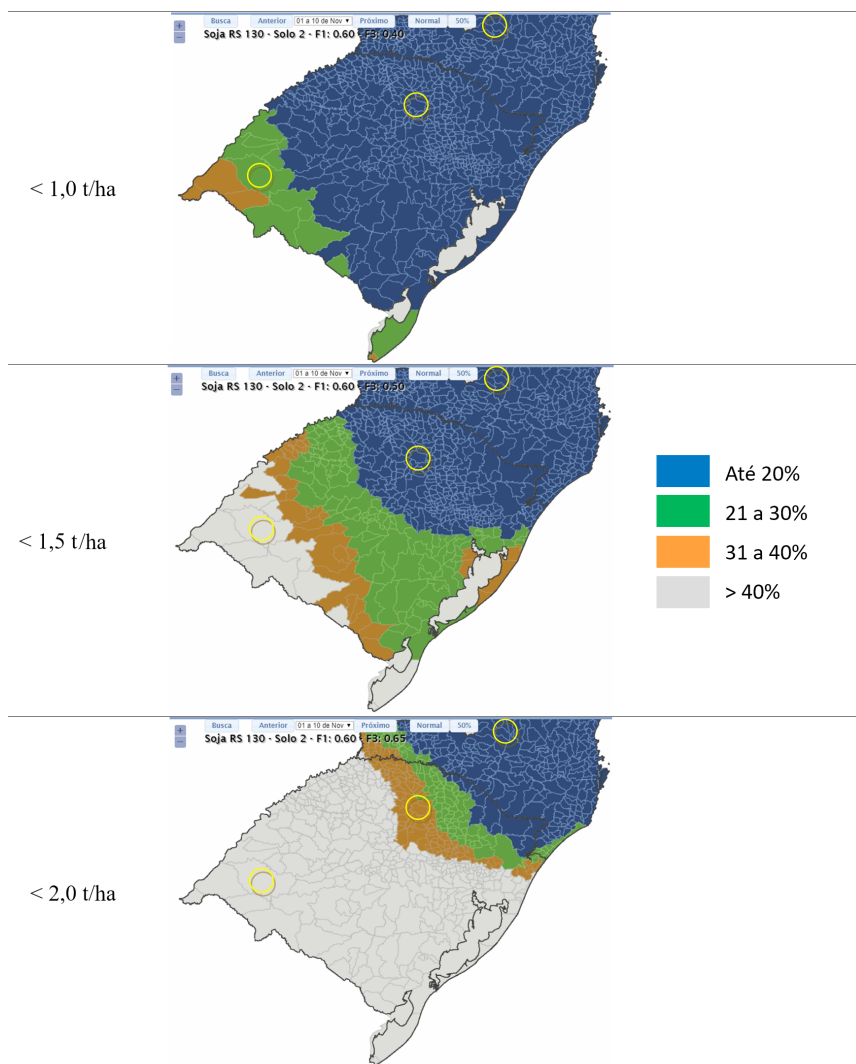
Figura 5. Zoneamento Agrícola de Risco da Produtividade Climática (ZARCPro) da soja no extremo sul do Brasil com 3 níveis de produtividade esperada e classes de risco de até 20%, 21 a 30%, 31 a 40% e maior que 40%. Os municípios de Irineópolis em Santa Catarina, Passo Fundo e Alegrete no Rio Grande do Sul encontram-se destacados pelos círculos sobre o mapa.
